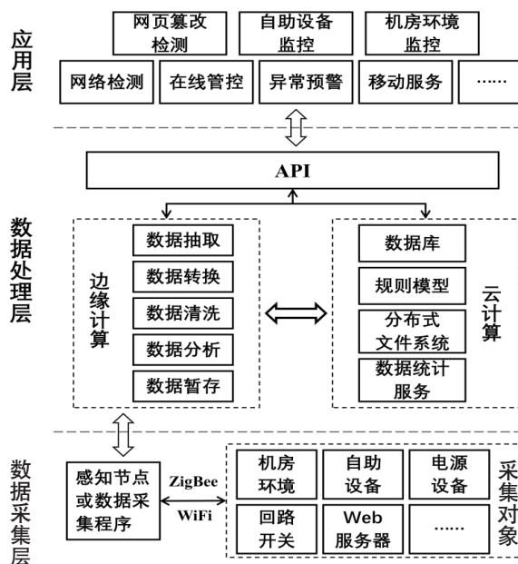
图1 系统架构
